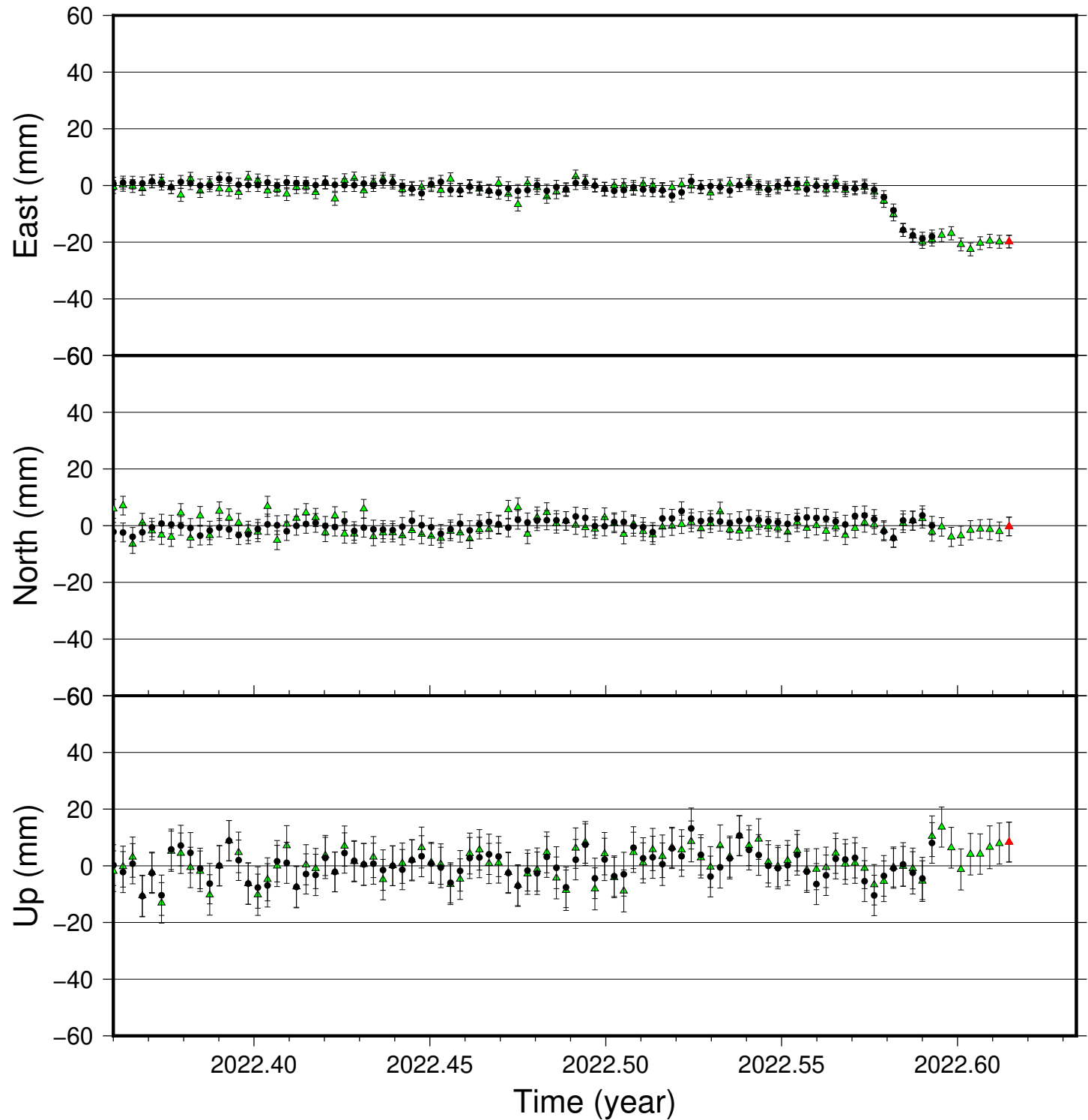
AFST time series (IGS 2014), last 100 days
